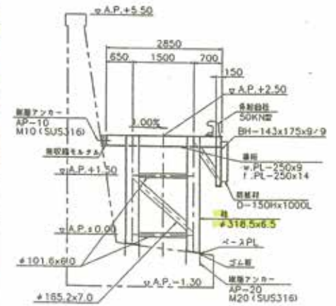
図3. 横橋断面図
